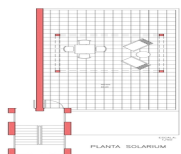
PLANTA SOLARIUM SUP. UTIL : 80,00 M2. SUP. CONSTRUIDA: 75,00 M2. SUP. DE TERRAZAS DESC.: 11,00 M2. SUP. DE CUBIERTA : 60,00 M2.
